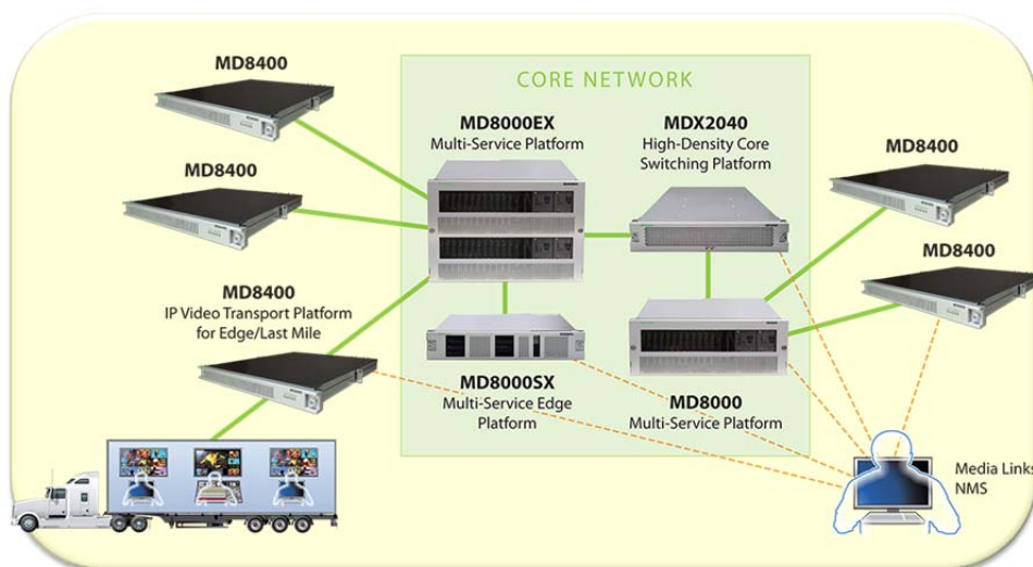
MD8000/MD8400 を用いたネットワークの構成イメージ
